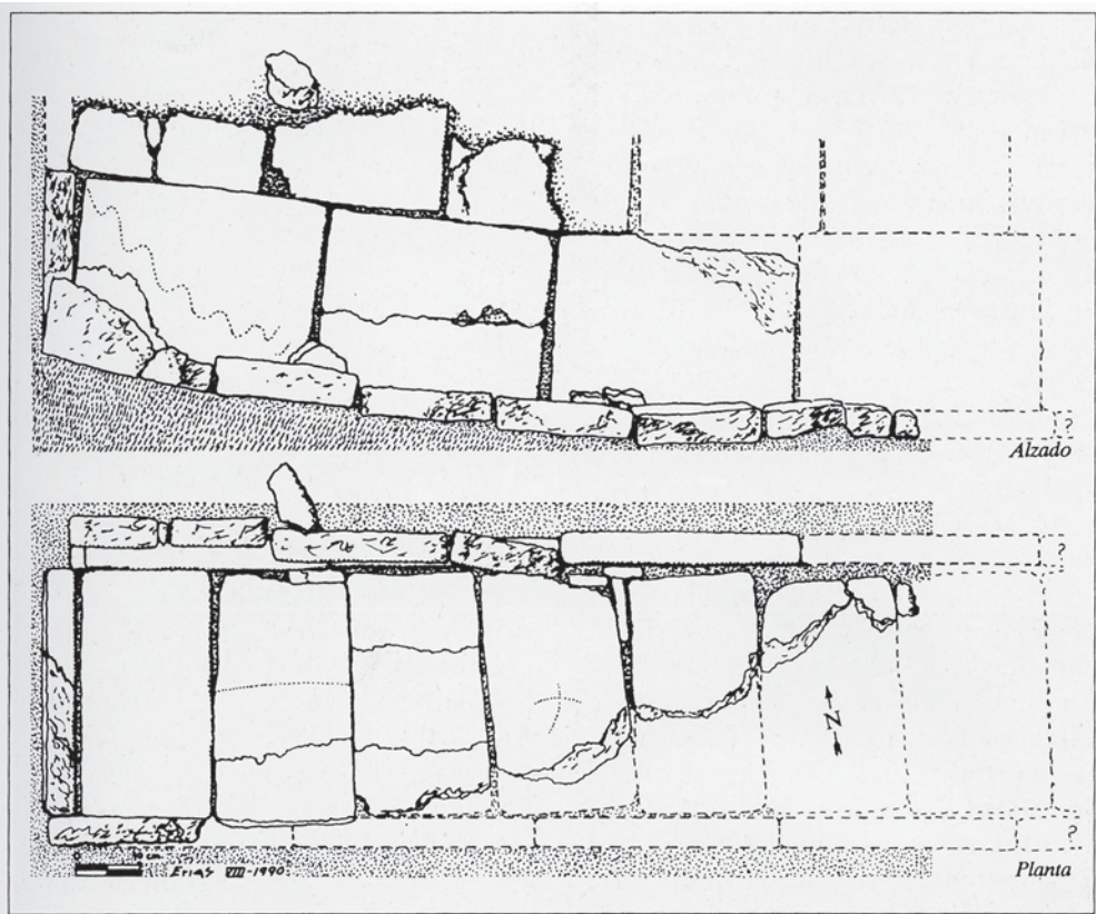
Planta e alzado do sepulcro tardorromano ou altomedieval de Paleo.
